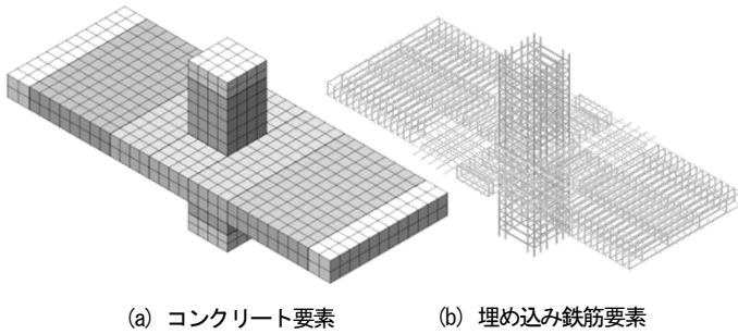
(a) コンクリート要素 (b) 埋め込み鉄筋要素 図 13 解析モデル形状
