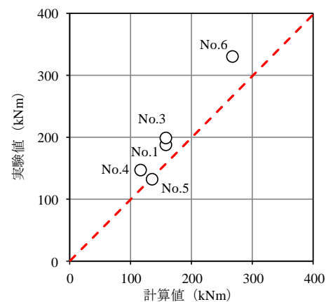
図12 終局曲げ耐力
