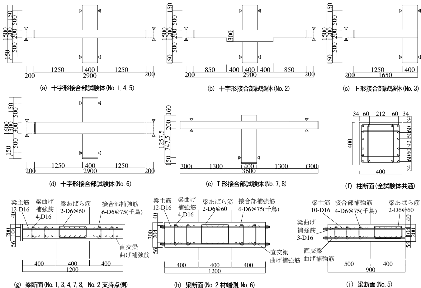
図2 試験体形状
