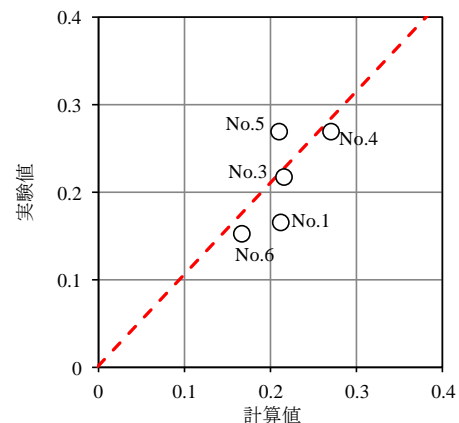
図11 降伏時剛性低下率
