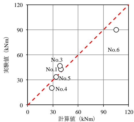
図10 曲げひび割れモーメント
