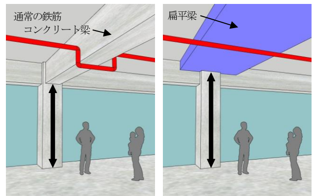
図 1 扁平梁による室内空間の有効利用例
