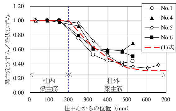
図 9 降伏ひずみで基準化した梁主筋ひずみの分布
