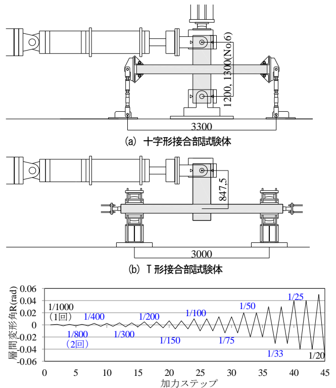
(c) 加力スケジュール 図 3 加力方法
